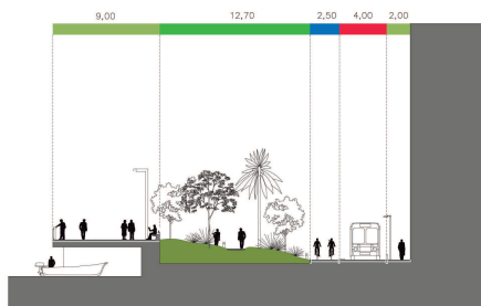
Sección transversal calle Rodríguez Sampedro (zona taller de embarcaciones)
